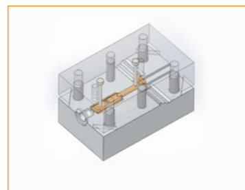
2. Konstruktion von Aluminiumformen in unserem eigenen Werkzeugbau
