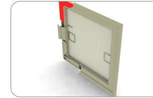
Eckkupplung für Profil mit Bördelung Innere
